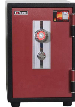
KF 35D OUT: W: 305 x D: 374 x H: 380 IN: W: 223 x D: 210 x H: 329
